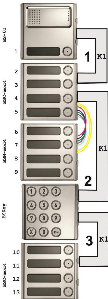
Obr. 3 Vzájemné propojení modulů Brave Steel
