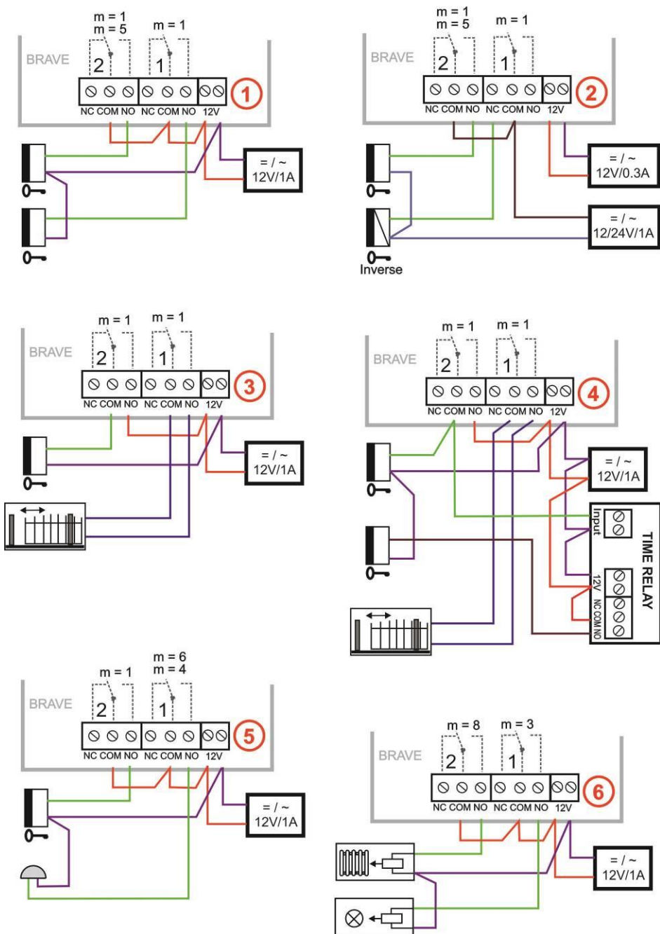
Obr. 4 Příklad zapojení spínačů
