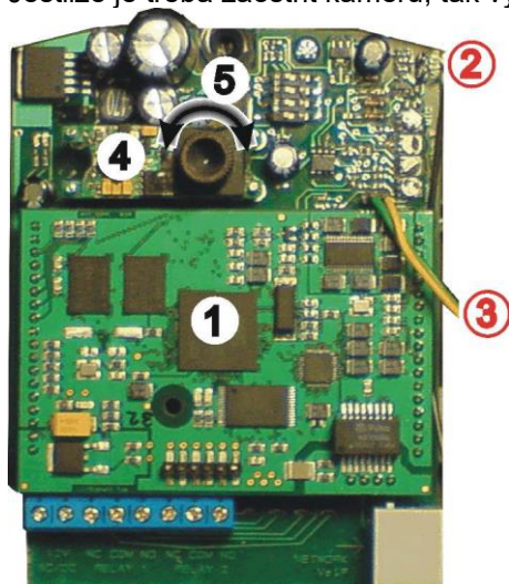
Obrázek 5 přední panel základního modulu IPDP
