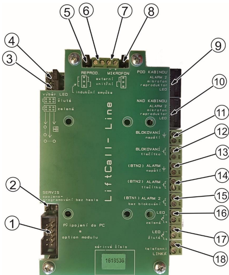
Picture 1: BraveLCL základní modul shora
